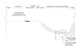
Secció transversal ST6: Secció constructiva en creuaments de carreteres o del tronc principal de vies de diversos carrils
