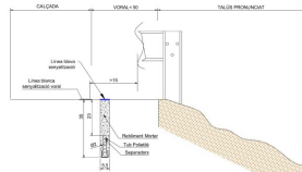
Secció transversal ST4: Secció constructiva de microrasa en presència de bona
