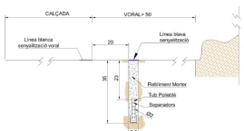
Secció transversal ST2a: Secció constructiva de microrasa en presència de cuneta transitable de formigó
