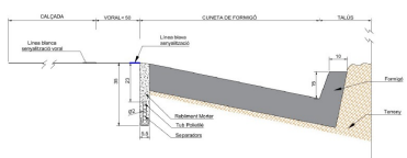
Secció transversal ST2a: Secció constructiva de microrasa en presència de cuneta transitable de formigó
