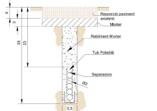
Secció transversal ST8: Secció constructiva de micro-rasa sota la vorera o rigola
