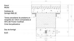
Canalització Convencional de 6c20 - EN VORERA
